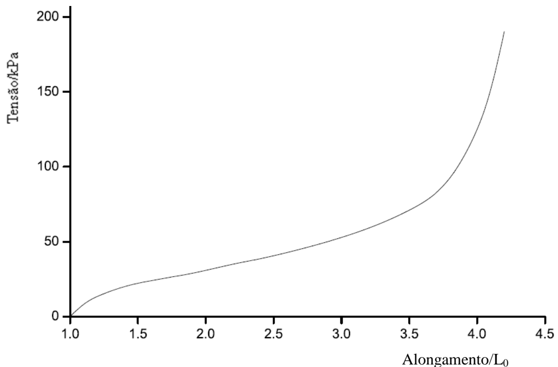
Figura 2. Curva típica de um ensaio de tração em uma borracha.
